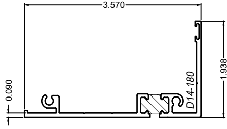
SUB-FRAME, 3-1/4" D14-180
